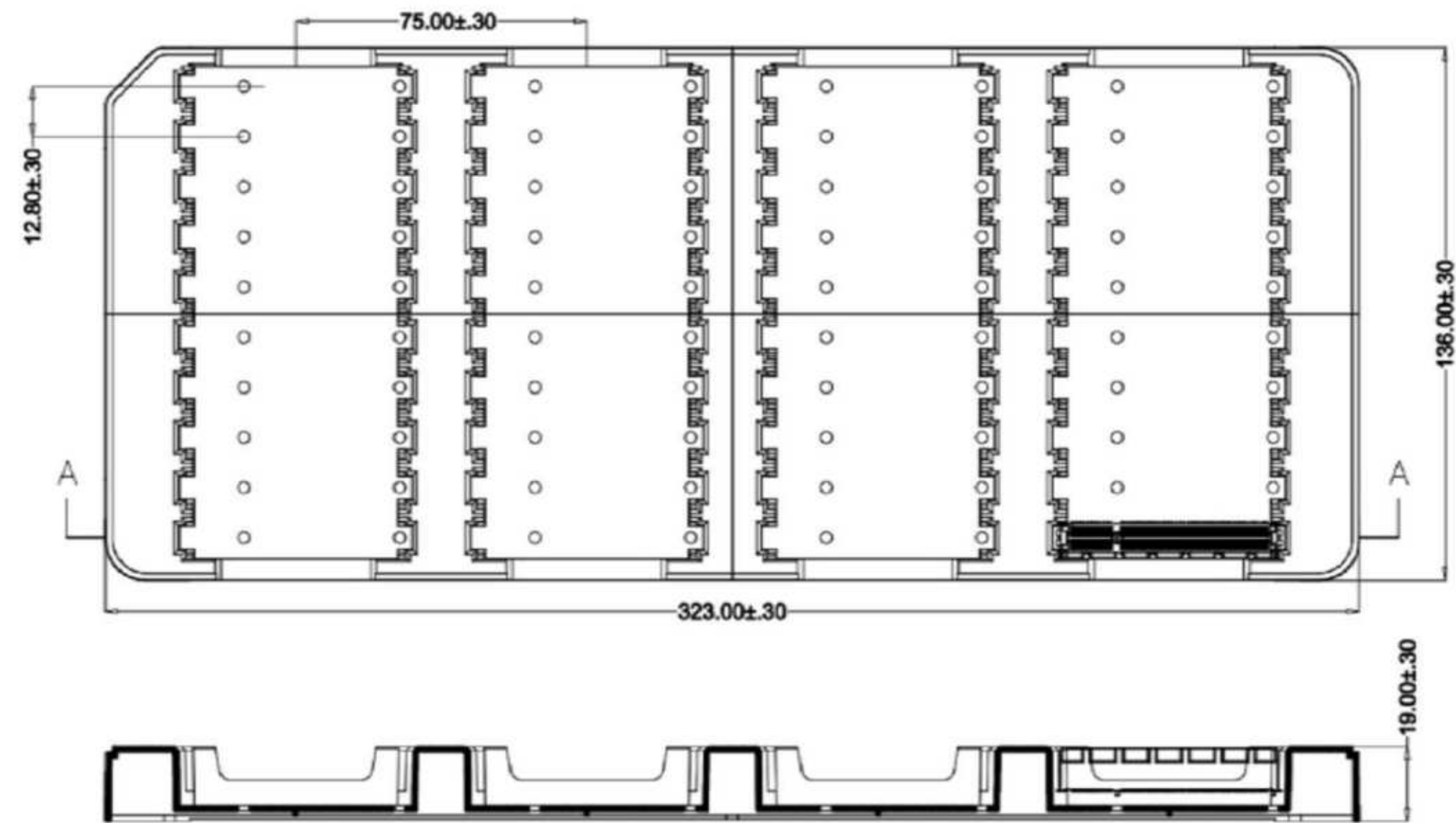
SECTION A-A
