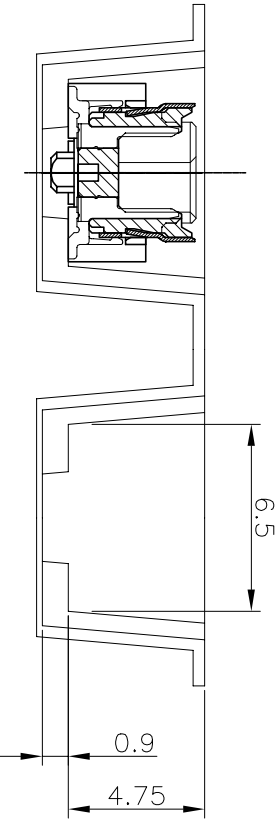
SECTION A-A SCALE 4:1
