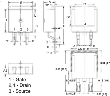
TO-263 Outline
