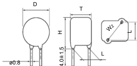
(ERZV10D182CS)
