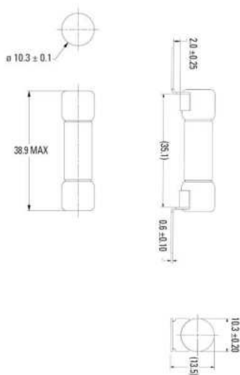
ZXBDB Bolt Down (Axial)
