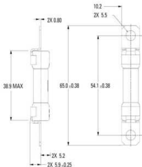
ZXBDB Bolt Down (Axial)
