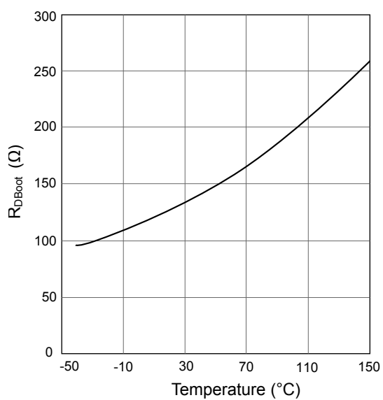
Figure 25. Typ R_{Dboot} vs. T_J
