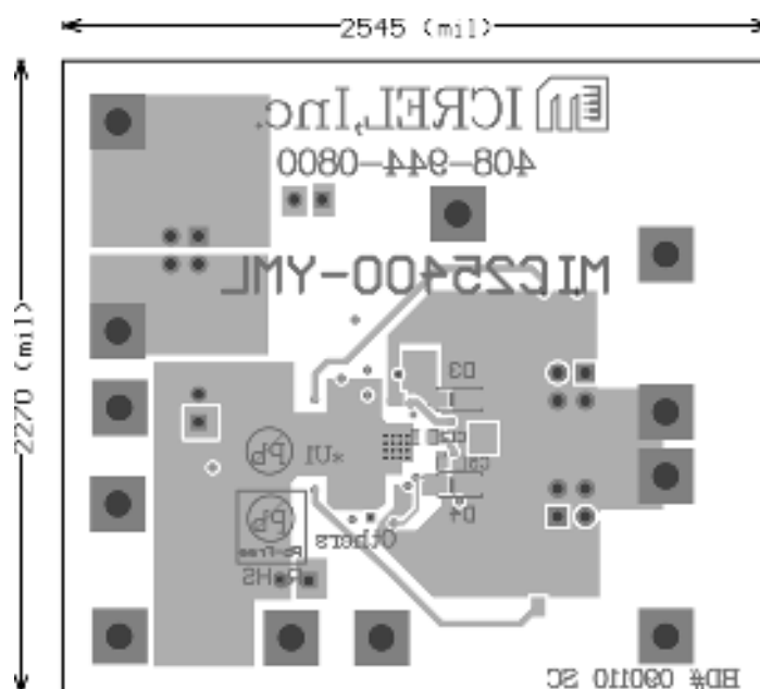
Bottom Layer
