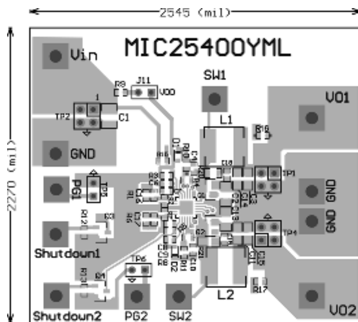
Top Layer
