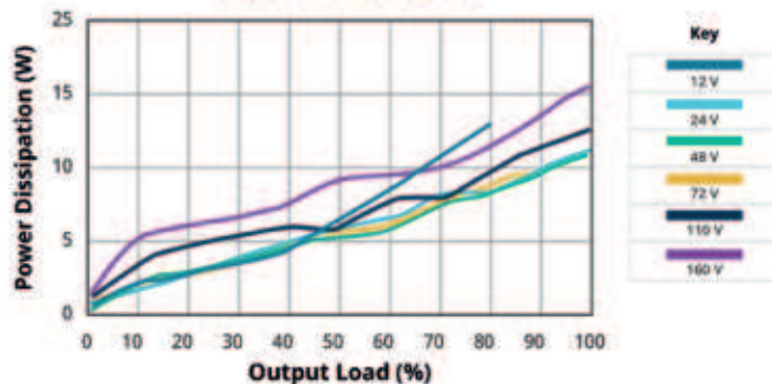
POWER DISSIPATION VS OUTPUT POWER 25°C PVQ100W-072-S24-D
