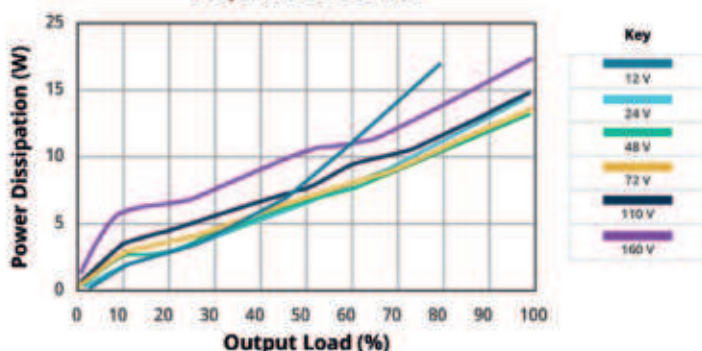
POWER DISSIPATION VS OUTPUT POWER 25°C PVQ100W-072-S12-D
