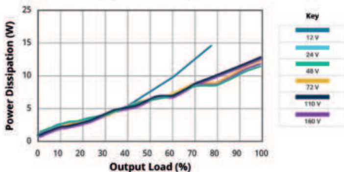
POWER DISSIPATION VS OUTPUT POWER 25°C PVQ100W-072-S15-D
