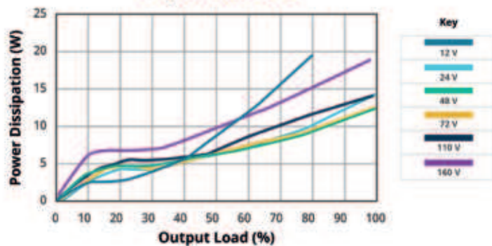
POWER DISSIPATION VS OUTPUT POWER 25°C PVQ100W-072-S5-D
