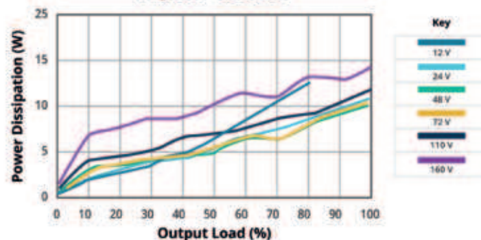
POWER DISSIPATION VS OUTPUT POWER 25°C PVQ100W-072-S28-D
