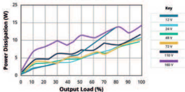
POWER DISSIPATION VS OUTPUT POWER 25°C PVQ100W-072-S54-D
