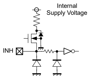
&lt;INH pin (R5110xxx2x)&gt;
