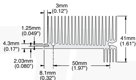
Clip Dimensions
