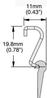
Clip Dimensions
