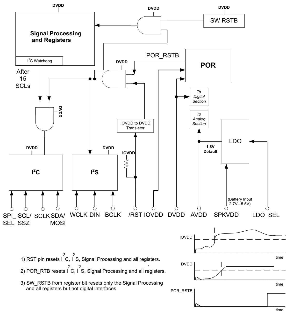
Figure 3-7. POR Diagram
