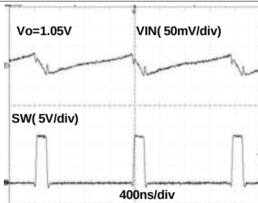
Figure 15. VIN Ripple
